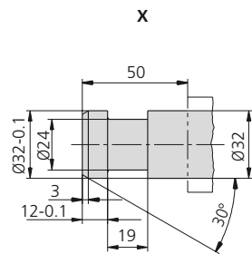
ejector bolt
